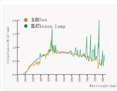
实验室光源与太阳光谱对比
