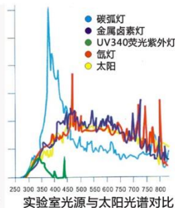
实验室光源与太阳光谱对比
